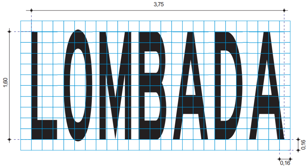
Figura 1- GABARITO LEGENDA "LOMBADA"
