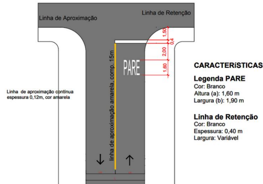
Figura 2- MODELO DO PARE COM FAIXA DE RETENÇÃO
